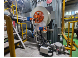
보일러 버너 개선 (저녹스 → 초저녹스)
